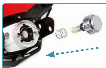
3 Insérer le ressort et la led
